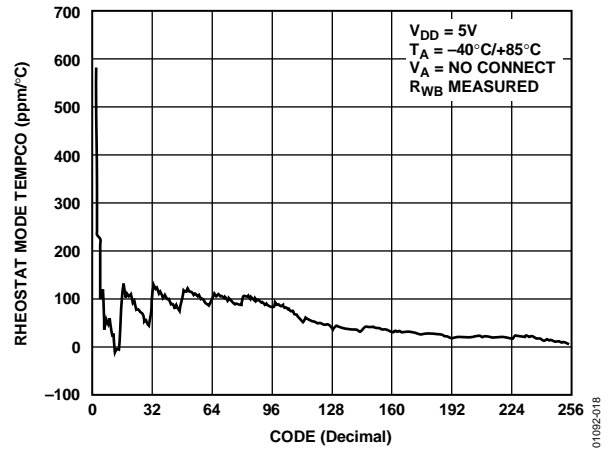
Figure 18. \Delta R_{WB}/\Delta T Rheostat Mode Tempo
